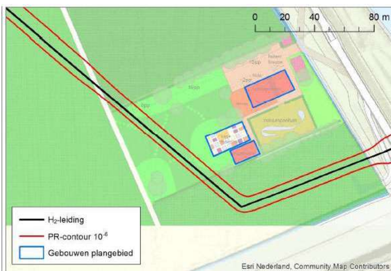
Figuur 4.4 Plaatsgebonden risicocontour 10^{-6} waterstofleiding (rode lijnen).
